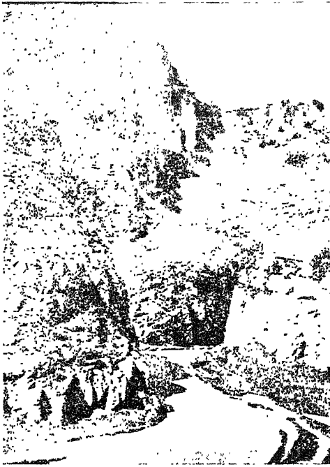
(अ) चेडार गाँज, समरसेट । कठोर कोयला युग की चूने की चट्टानों कुछ स्थानों पर सीधी व सुन्दर क्लिफ ४०० फीट ऊँची बनाती हैं ।
